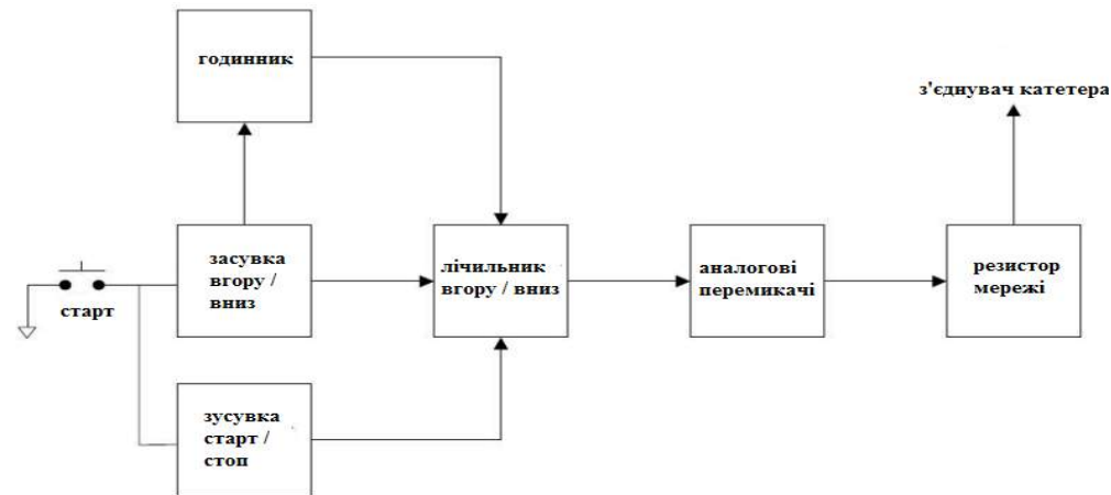
Рисунок 1 – Блок-схема імітатора US 7,998,082 B2
