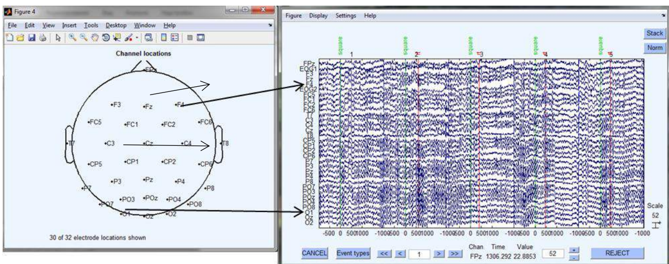
Рисунок 1 – Енцефалограма в програмі EEGLAB
