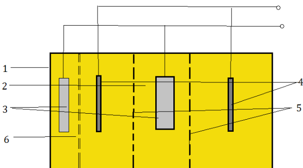
Рисунок 1. Схема мембранного електролізера.
