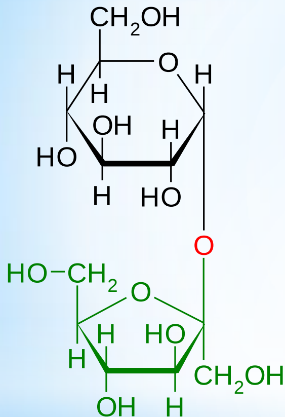
\beta -D-фруктофуранозил- \alpha -D-глюкопиранозид
