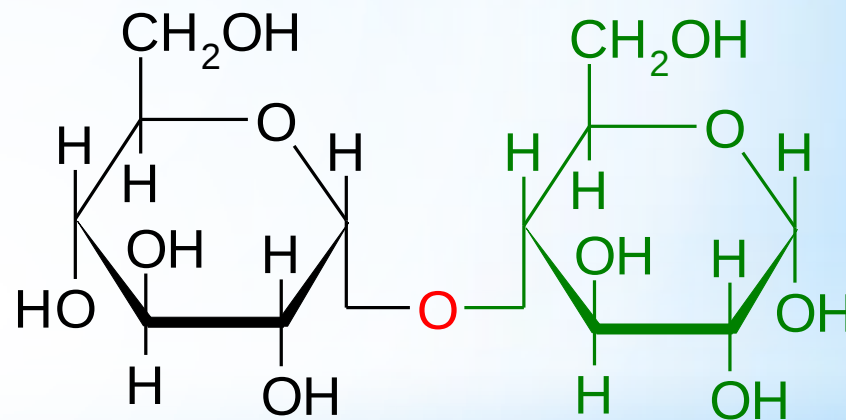
\alpha -D-глюкопиранозил-(1 \rightarrow 4)- \alpha -D-глюкопираноза
