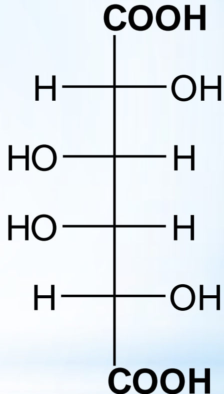
галактаровая кислота
