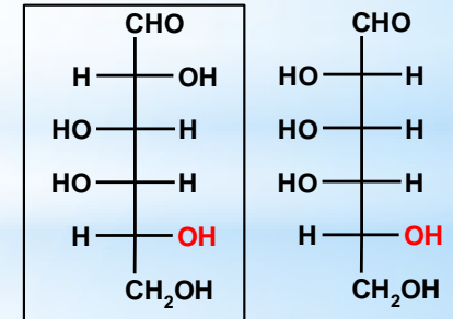
D-галактоза D-галола
