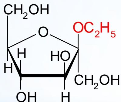
O-этил-β-D-фруктофуранозид
