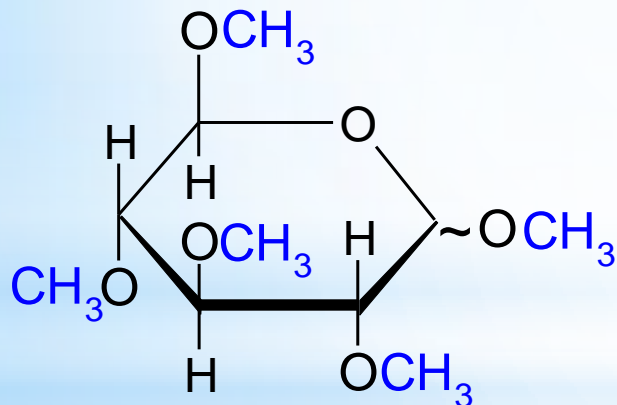
O-метил-2,3,4,6-тетраметил-D-глюкопиранозид
