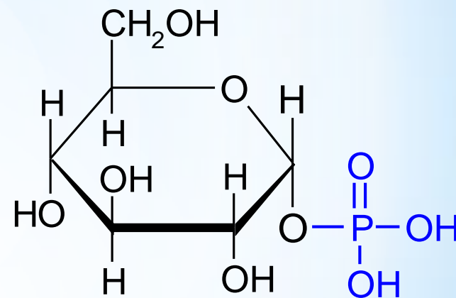
D-глюкозо-1-фосфат
