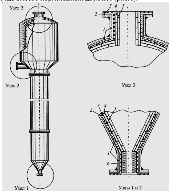
Рисунок 1 – Схема антикоррозионной защиты гидратора ацетилена: 1 – углеродистая сталь; 2 – клеевая прослойка; 3 – полиизобутилен ПСГ или резина на основе НК; 4 – кислотоупорная замазка; 5 – кислотоупорная плитка; 6 – патрубок из плавяного диабаз, фарфора или ситалла
