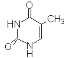
Тимин (Т) (5-метил-2,4-диоксопиримидин)
