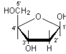
2-Дезокси- \beta -D-рибофураноз
