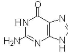
Гуанин (Г) (2-амино-6-оксопурин)
