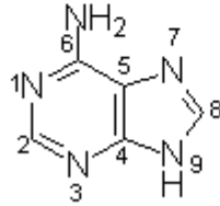
Аденин (А) (6-аминопурин)
