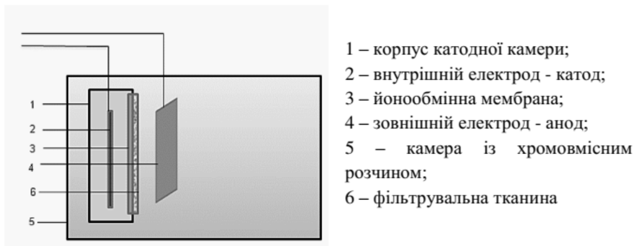
Рисунок 1 – Схема мембранного електролізера із зовнішнім анодом
