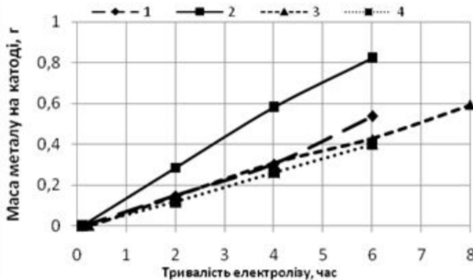
Рисунок 1. Вплив перемішування на електровідновлення металів на катоді при їх міграції через катіонообмінну мембрану при температурі електроліту 20 °С 1 -аноліт з перемішуванням, містить \text{Cd}^{2+} ; 2 -аноліт без перемішування, містить йони \text{Cd}^{2+} ; 3 -аноліт без перемішування, містить йони \text{Zn}^{2+} , 4 -аноліт з перемішуванням, містить йони \text{Zn}^{2+}
