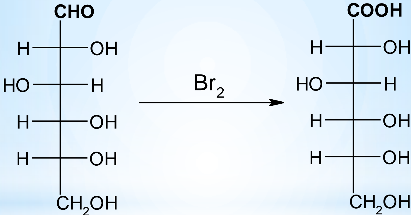
глюкоза
