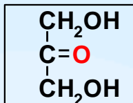
дигидроксиацетон
