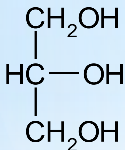
глицерин
