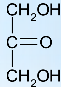
дигидроксиацетон
