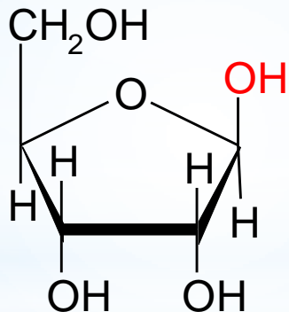
\beta -D-рибофураноза
