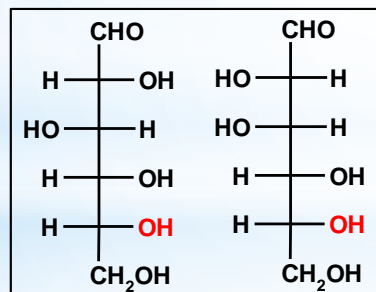
D-глюкоза
