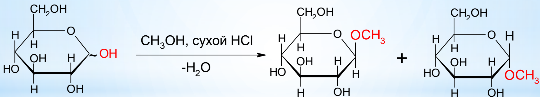
D-глюкопираноза
