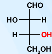
D-треоза
