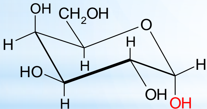
\alpha -D-галактопираноза
