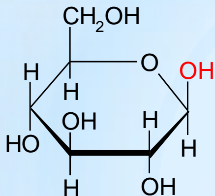
\beta -D-глюкопираноза
