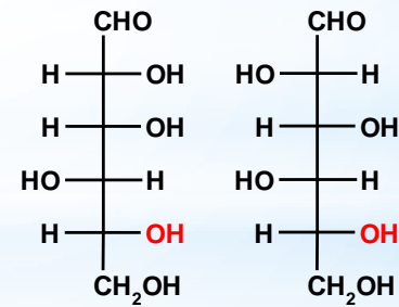
D-гулоза
