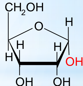
\alpha -D-рибофураноза
