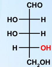
D-Ликсоза
