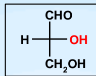
D-глицериновый альдегид
