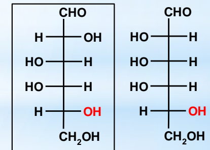
D-галактоза
