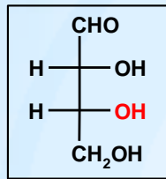
D-эритроза
