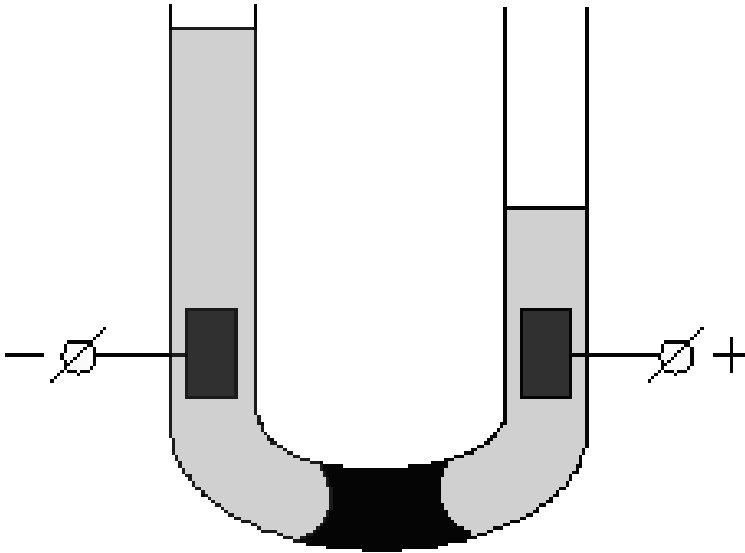
Рис. 6 Схема досвіду по електроосмосу
