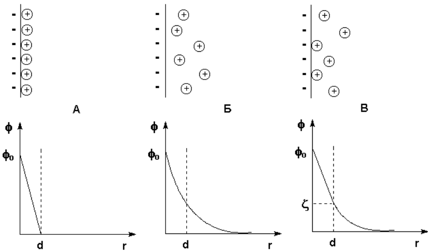
Рис. 4 Будова ДЕШ:
