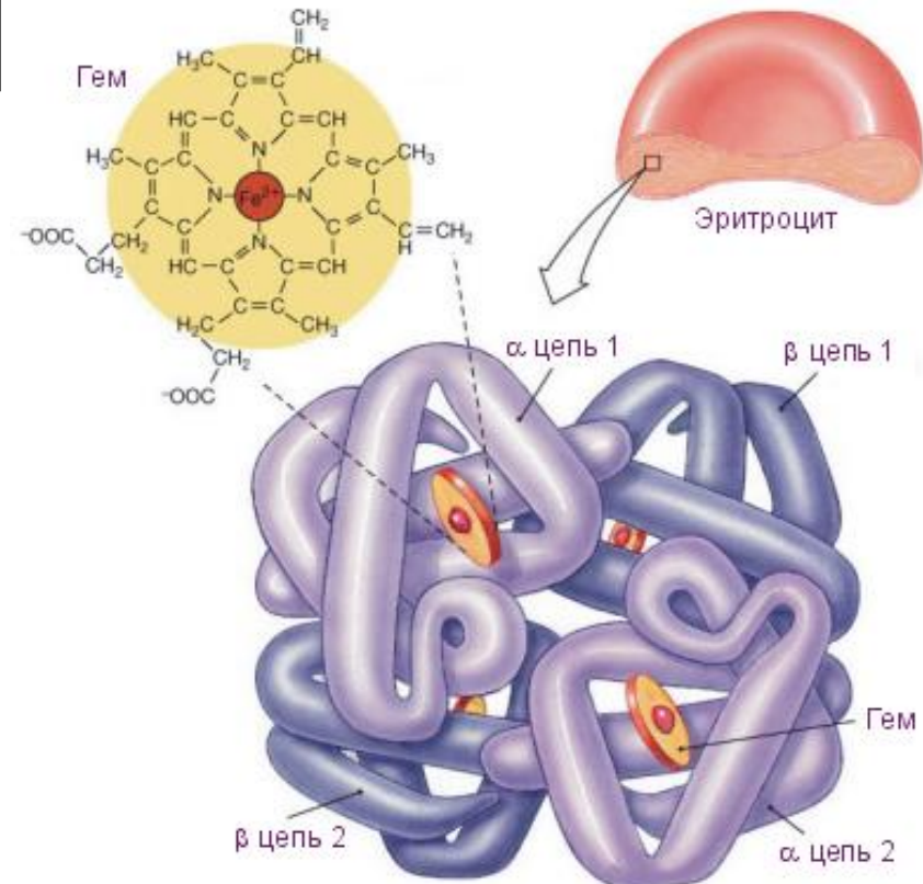
Молекула гемоглобіна
