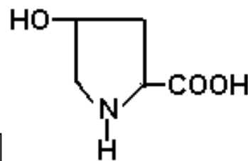
Оксихролін
