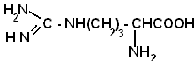
Аргінін
