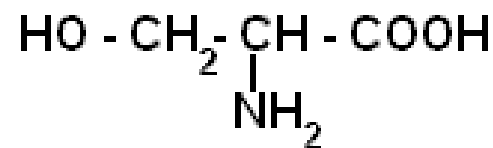
серин
