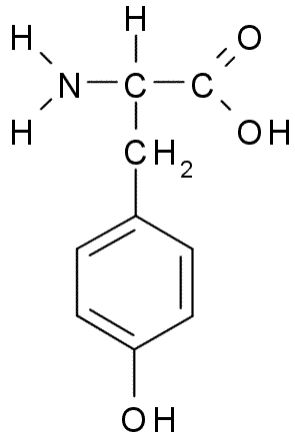
тирозин
